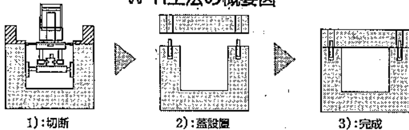
W2R工法の概要図
